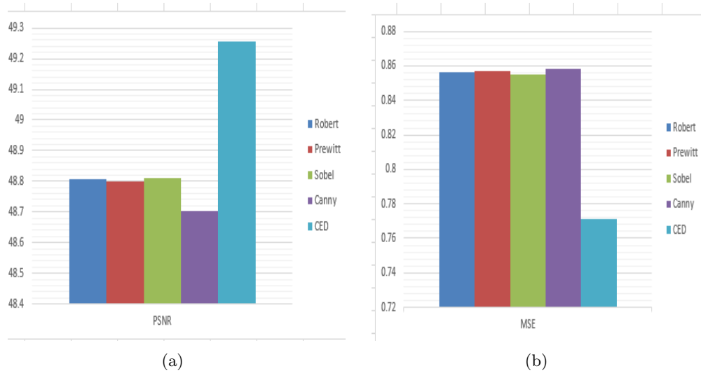
Figure 9: Result analysis of Dídà Olójúmèta
